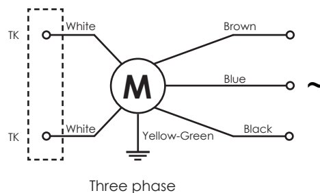
Motor wiring
